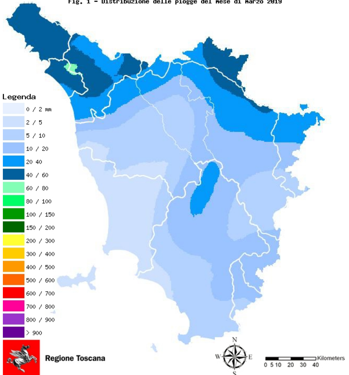
Fig. 1 - Distribuzione delle piogge del mese di marzo 2019
