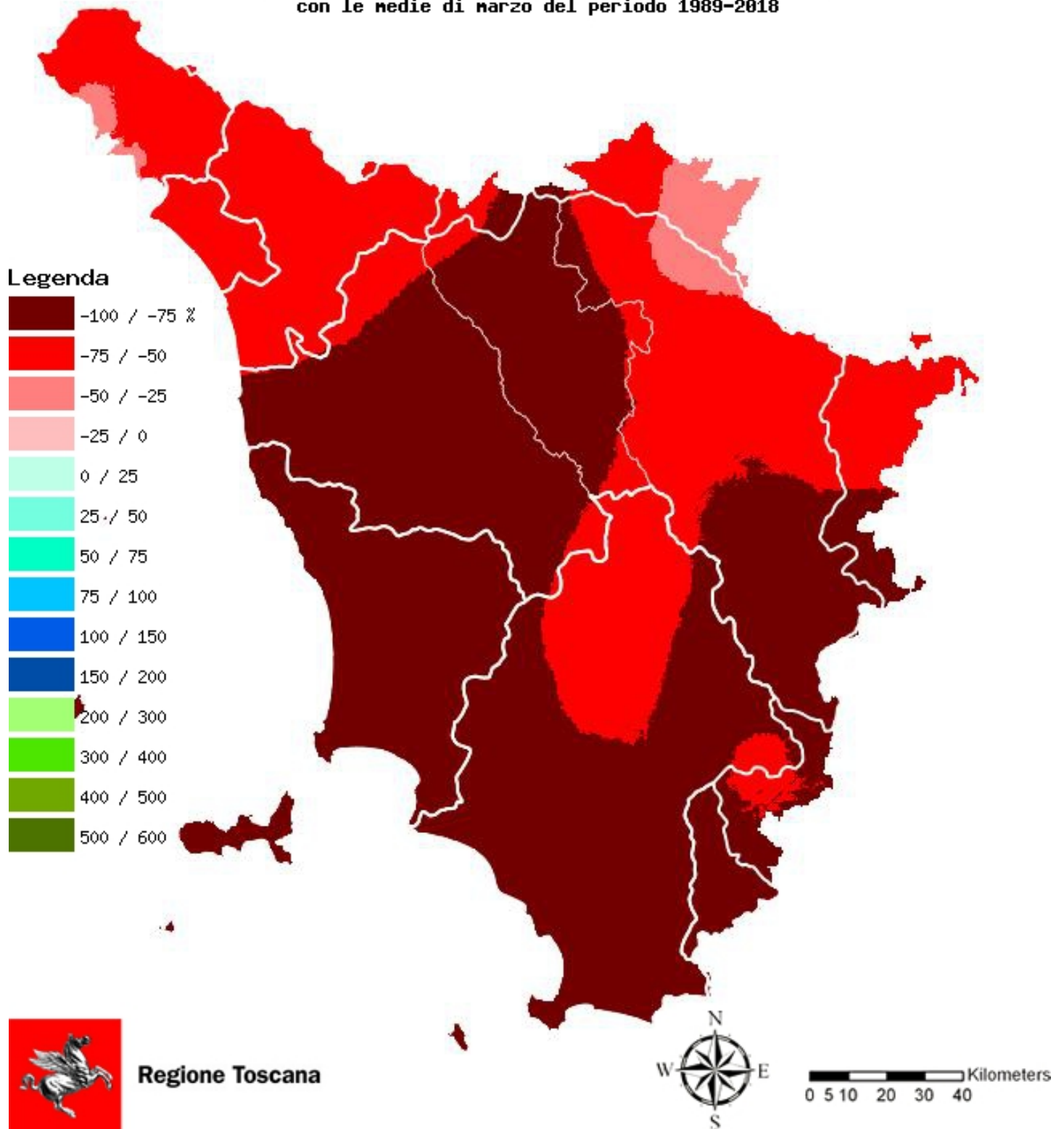
Fig. 2 - Confronto tra le precipitazioni (%) di marzo 2019 con le medie di marzo del periodo 1989-2018
