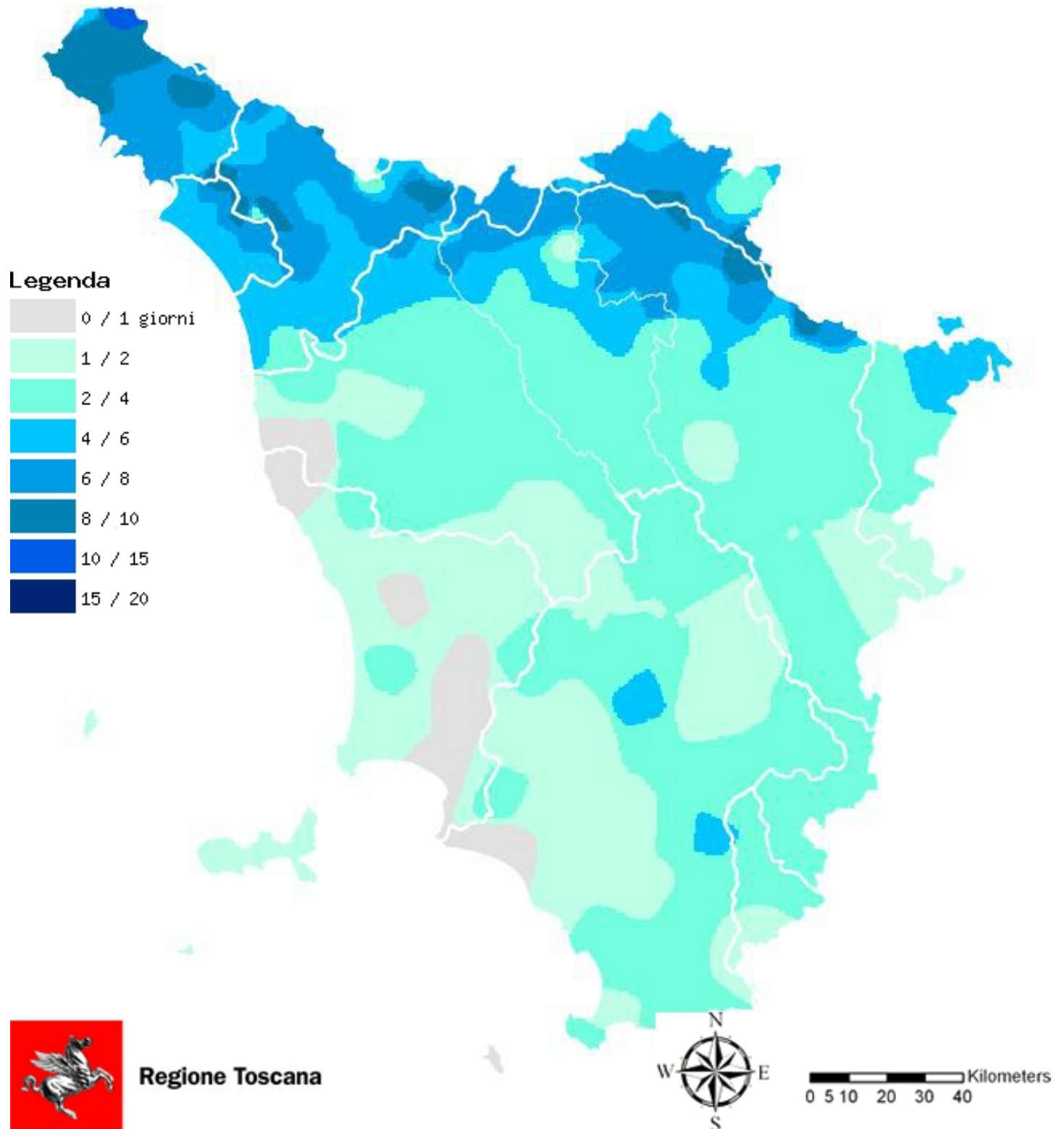
Fig. 4 - Distribuzione dei giorni piovosi ( \geq 1\text{mm} ) del mese di marzo 2019
